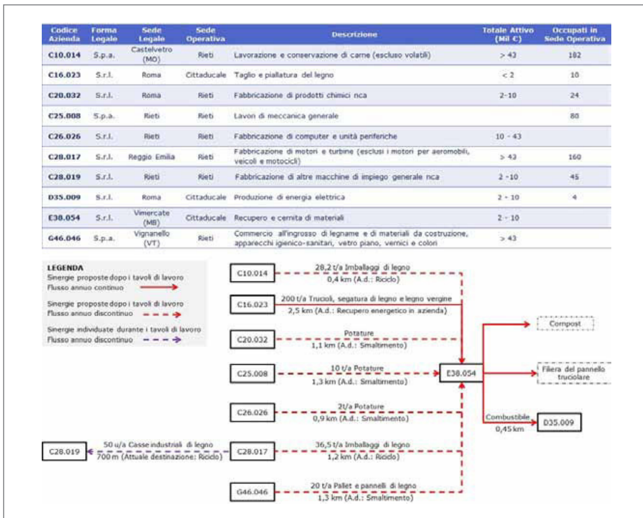
Fig. 1 Il possibile scenario di un ecosistema industriale nell'ASI di Rieti-Cittaducale Fonte: [6]
